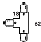
(G) Connexion T externe-droite Noir 6418060
