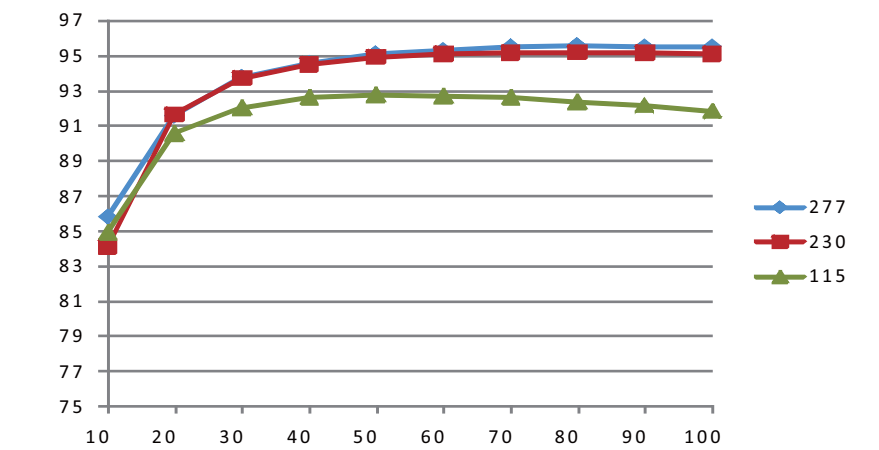
Rendement, en pourcentage, en fonction de la charge. Relevé sur le modèle 48 V de la gamme, température de boîtier à 80°C. Le rendement atteint jusqu'à 95 % en application.
