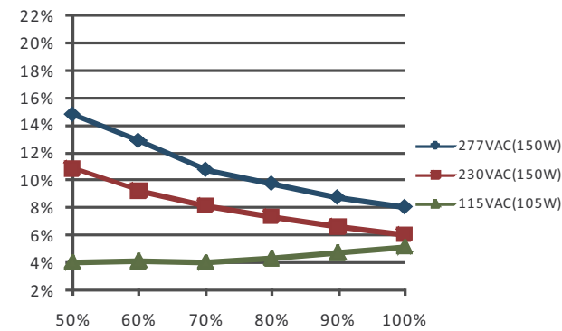
Distorsion harmonique totale, en pourcentage, en fonction de la charge. Relevé sur le modèle 54 V de la gamme, température de boîtier à 80°C.
