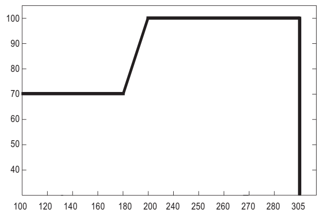
Charge admissible, en pourcentage de la puissance nominale, en fonction de la tension d'entrée en volts, à 60 Hz. Un déclassement est nécessaire sous faible tension d'entrée.
