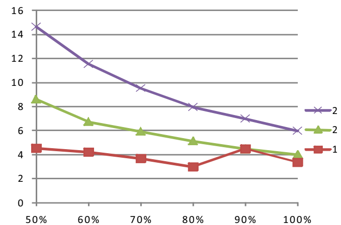
Distorsion harmonique totale, en pourcentage, en fonction de la charge. Relevé sur le modèle 48 V de la gamme, température de boîtier à 80°C.
