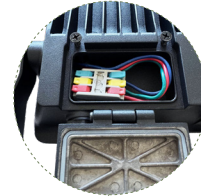
Raccordement direct du câble mural dans le bornier intégré au dos du projecteur
